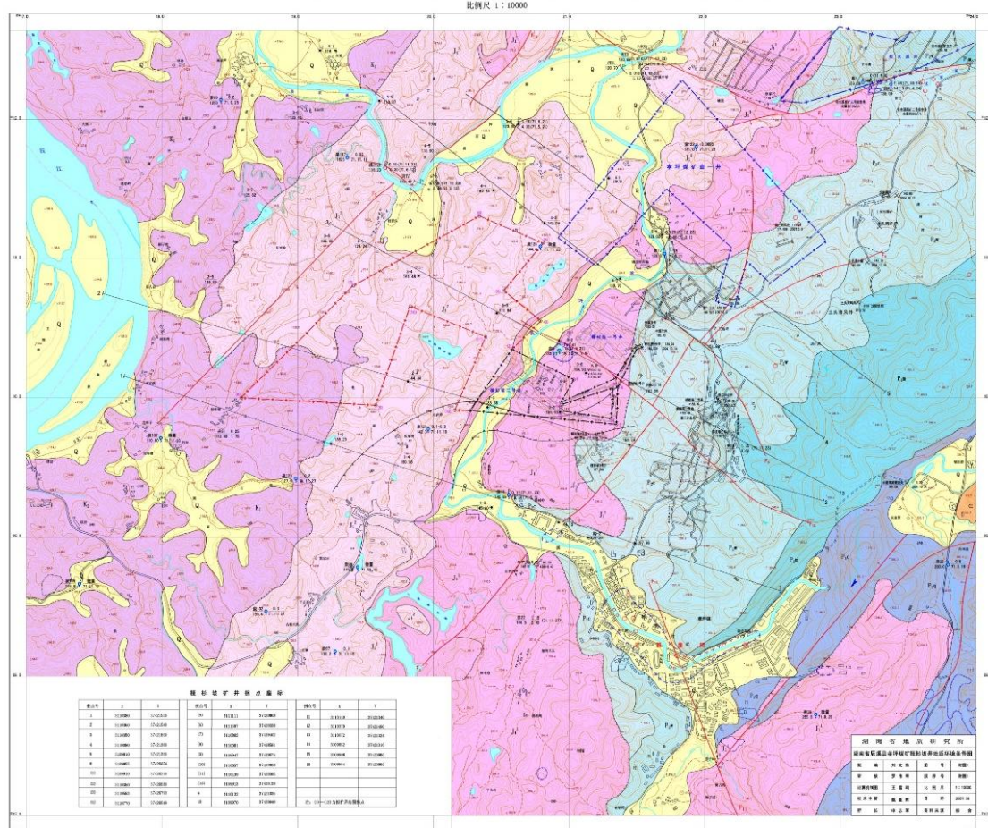
湖南省辰溪县孝坪煤矿桧杉坡井地质环境条件图
