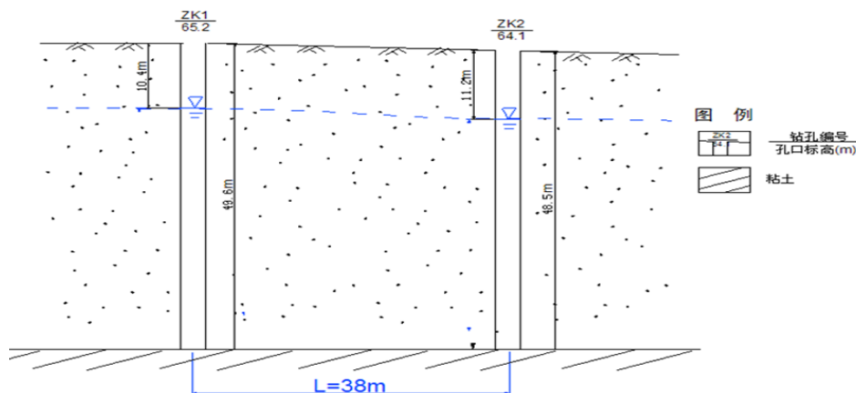
资料：某剖面线水文地质剖面图
